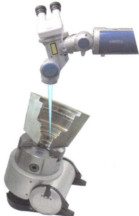
Laserschweißen in der Vertiefung Fokussierobjektiv 300 mm
